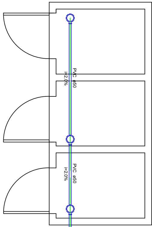
SUMIDOURO PLANTA BAIXA - ESC. 1:25
