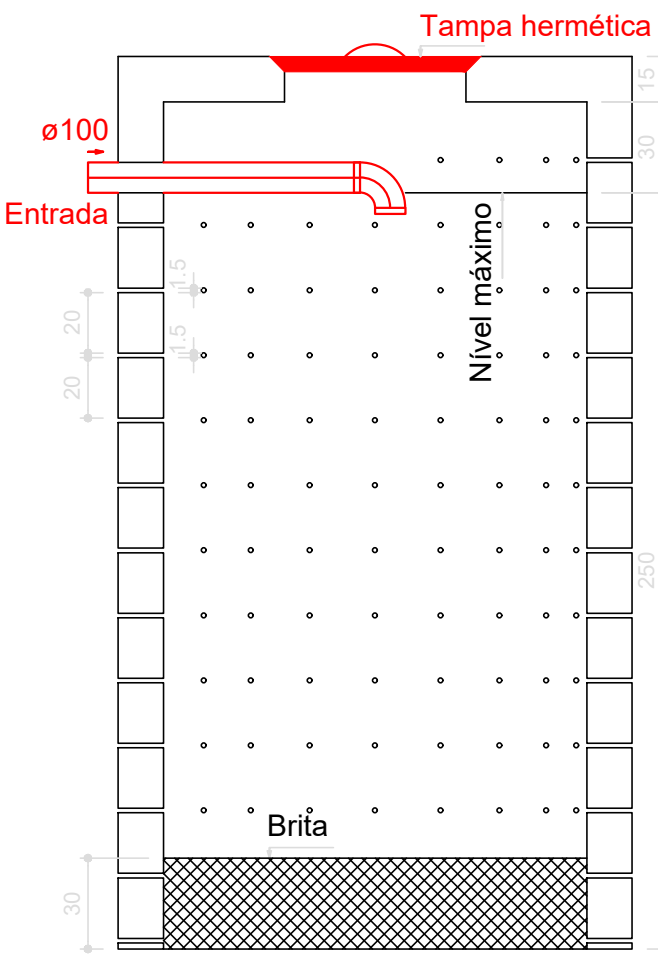
SUMIDOURO CORTE - ESC. 1:25
