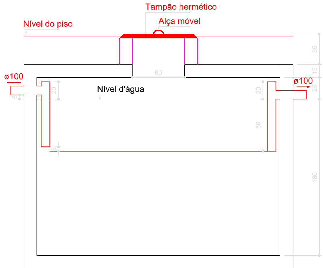
TANQUE SÉPTICO CORTE - ESC. 1:25
