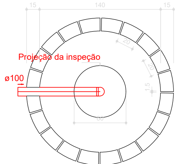
SUMIDOURO PLANTA BAIXA - ESC. 1:25
