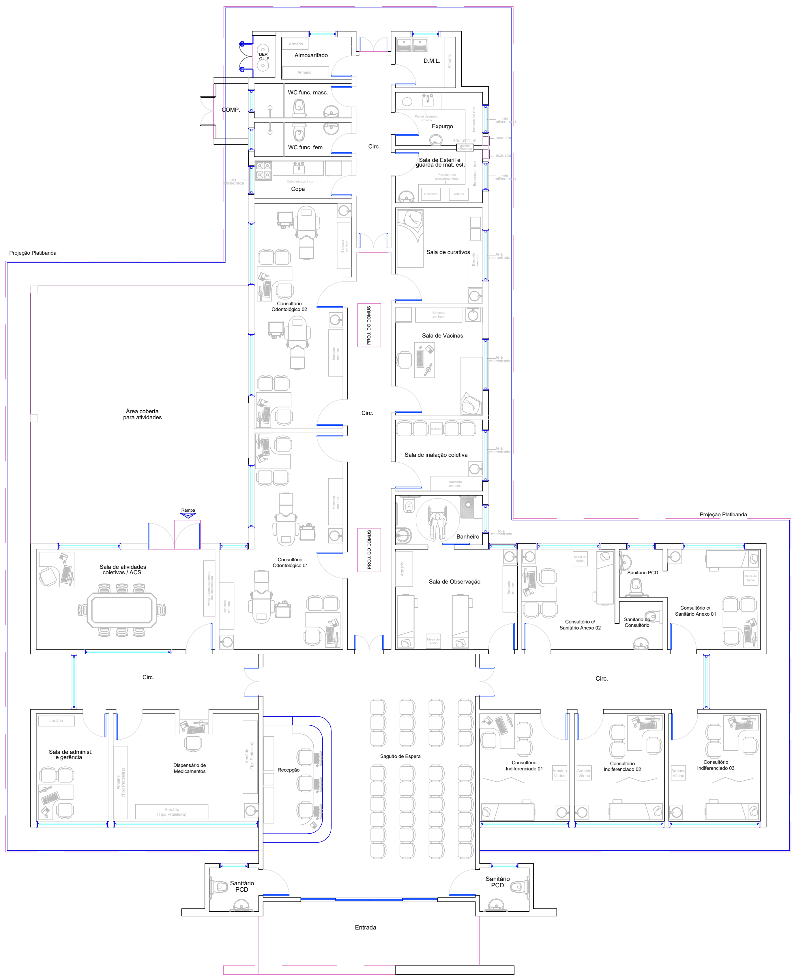
LAY-OUT 1:75
